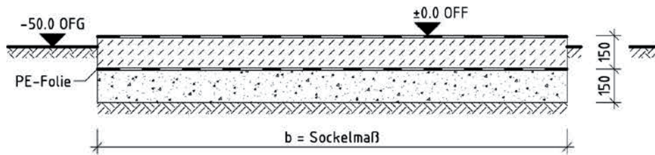
Schnitt A-B
